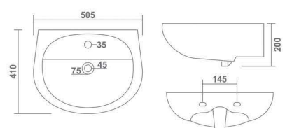
BLANCO L 505 W 410 H 200 mm 20" x 16"
