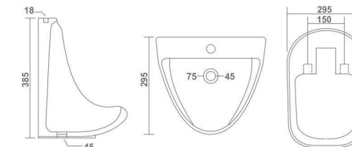
BABY L 295 W 295 H 385 mm
