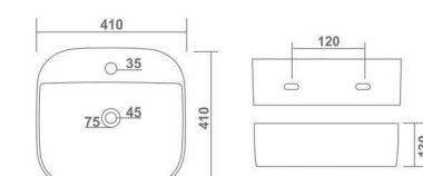
DELL L 410 W 410 H 130 mm 16" x 16"
