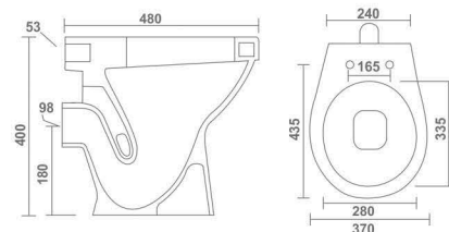
E.W.C. L 480 W 370 H 400 mm 'P' Trap
