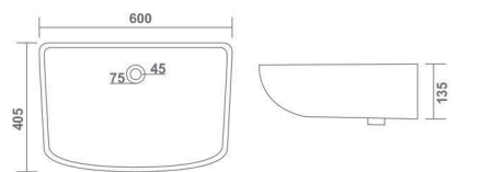
GRACIA L 600 W 405 H 135 mm 24" x 16"
