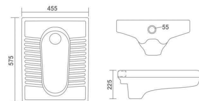
ORISSA PAN - 23" L 575 W 455 H 225 mm
