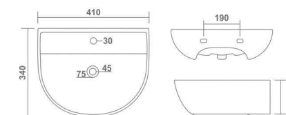
RIO L 410 W 340 H 165 mm 16" x 13"
