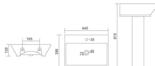
LUMINA L 445 W 390 H 815 mm 18" x 16"
