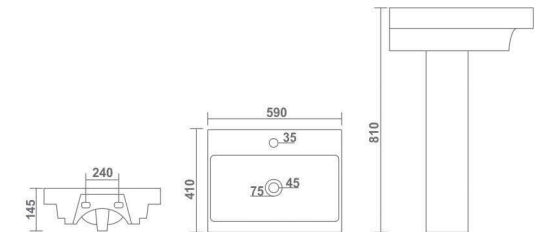
RIPPLE L 590 W 410 H 810 mm 24" x 16"
