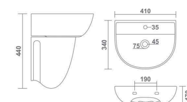
RIO L 410 W 340 H 440 mm 16" x 13"
