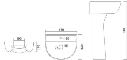
RIO L 410 W 340 H 840 mm 16" x 13"
